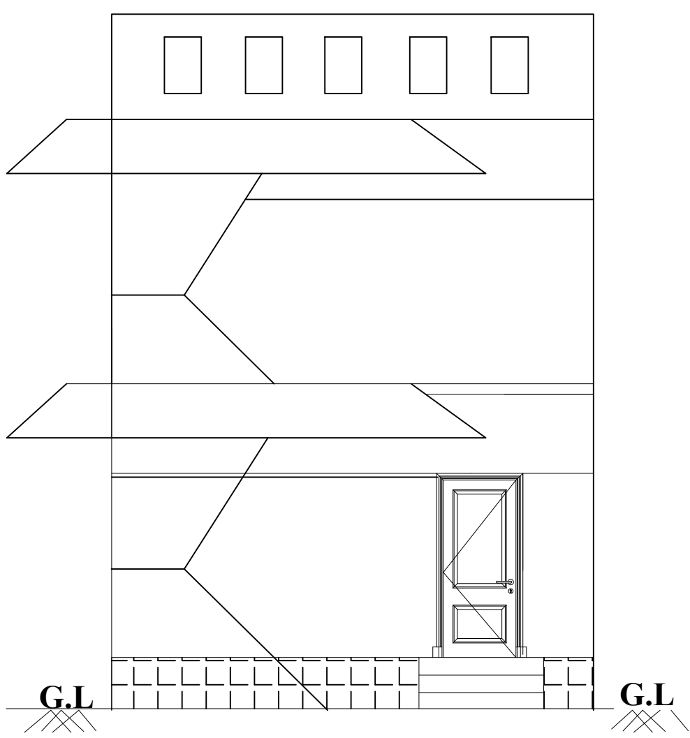
ELEVATION
