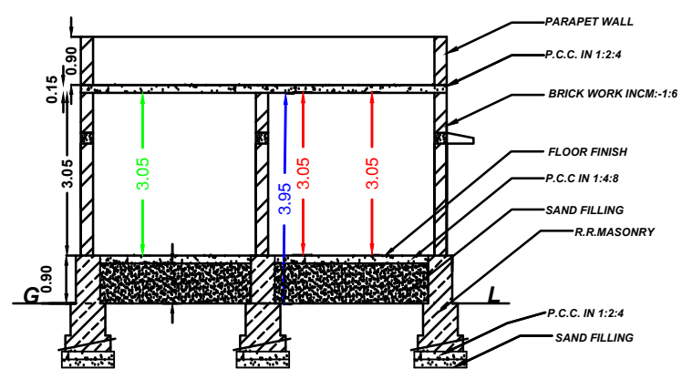
SECTION - AB
