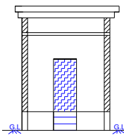
ELEVATION
