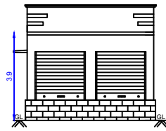
ELEVATION
