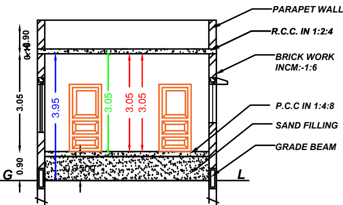
SECTION - AB
