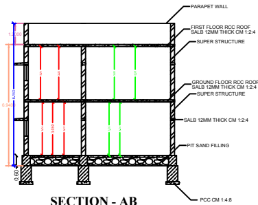
SECTION - AB
