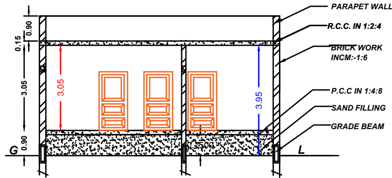
SECTION - AB
