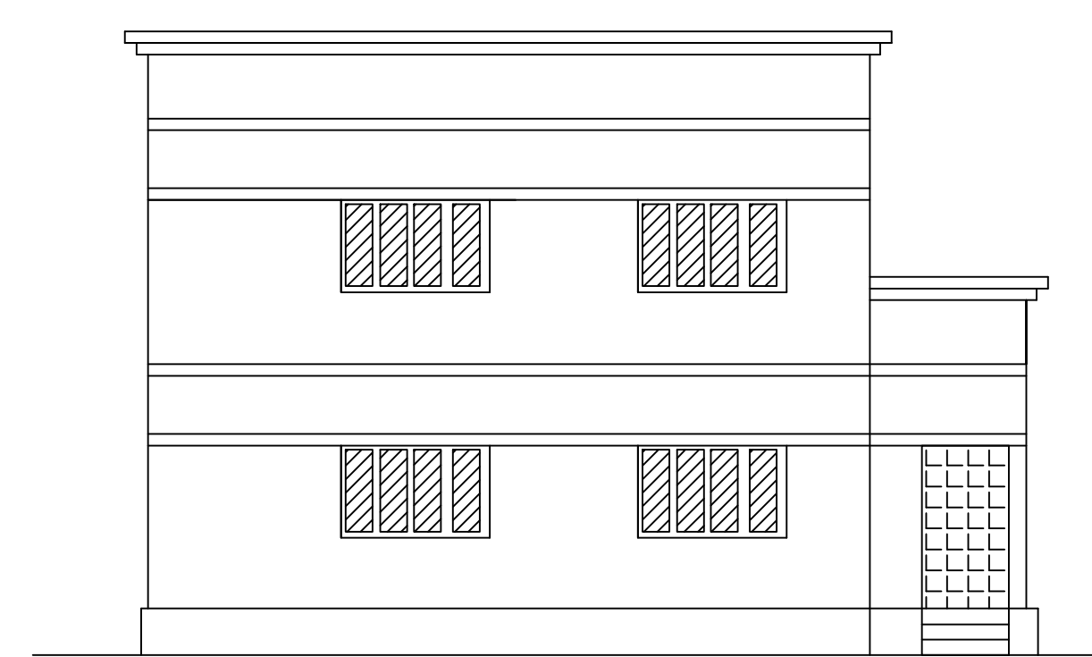
ELEVATION
