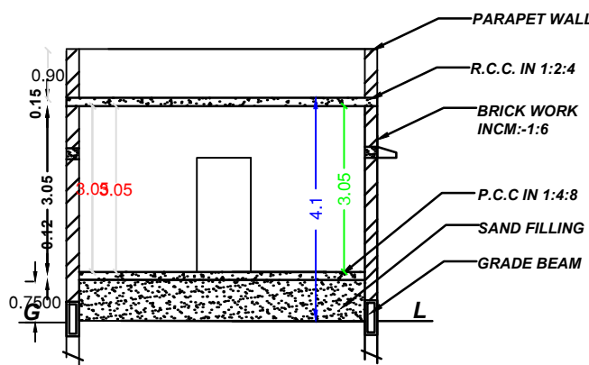
SECTION - AB
