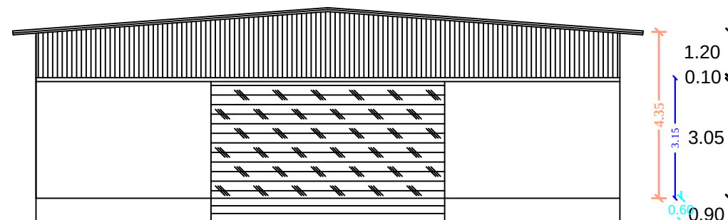
ELEVATION
