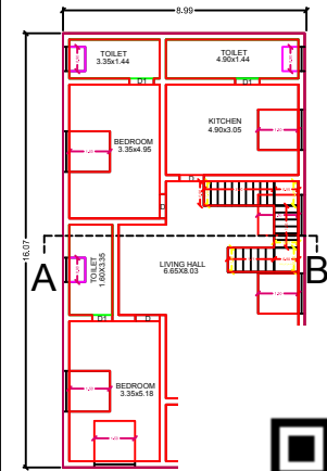
PLAN - GRC
