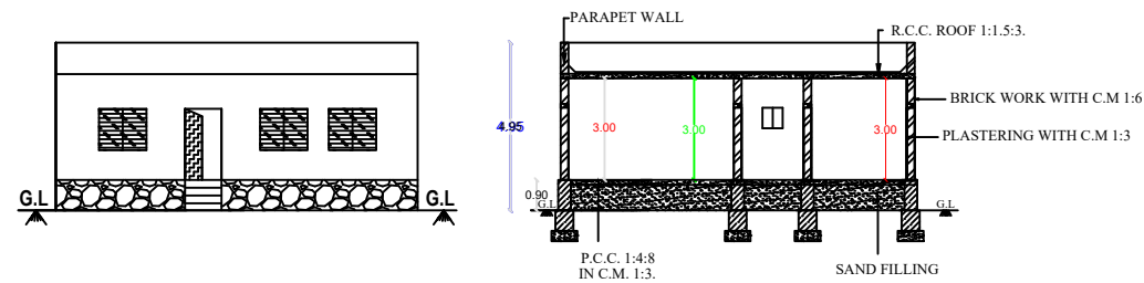
ELEVATION
