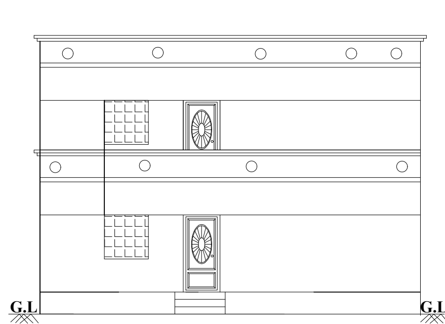
ELEVATION
