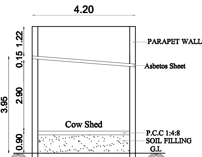
SECTION-A
