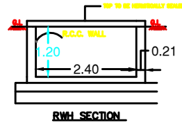
R.W.H. SECTION
