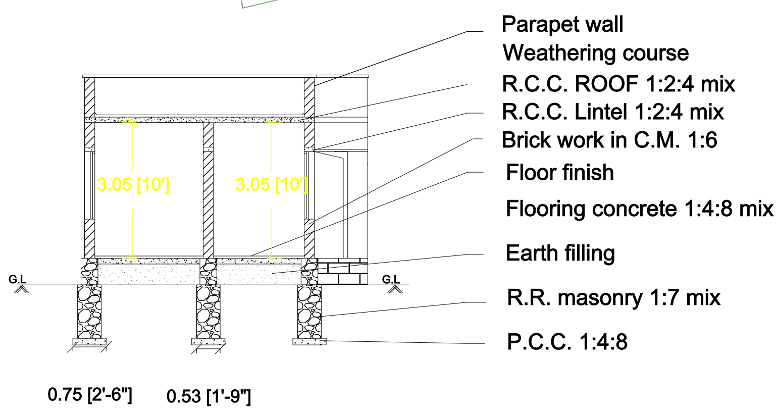
SECTION - AB
