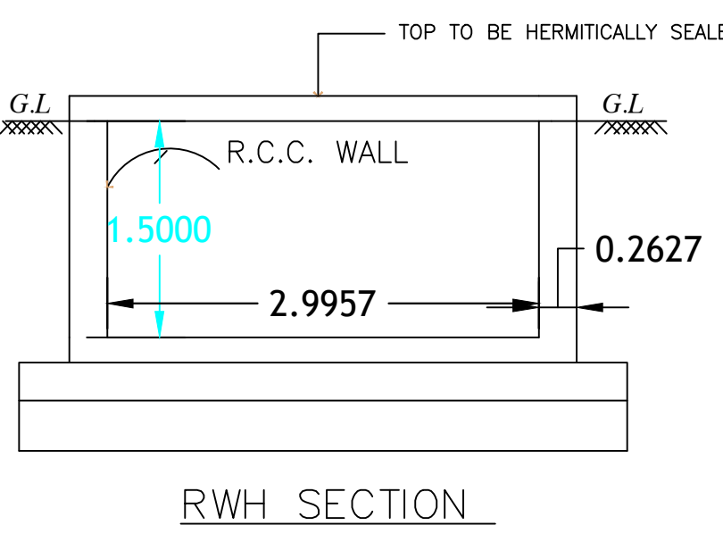
R.W.H. SECTION
