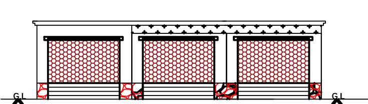
ELEVATION
