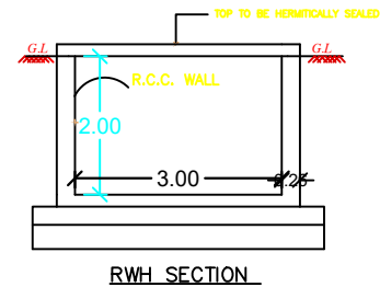
RWK SECTION
