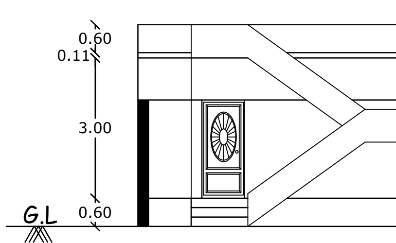
ELEVATION
