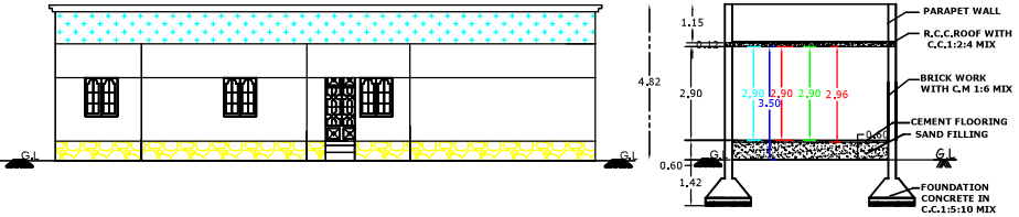
ELEVATION
