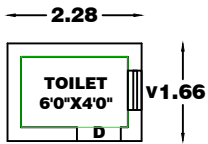
TOILET PLAN
