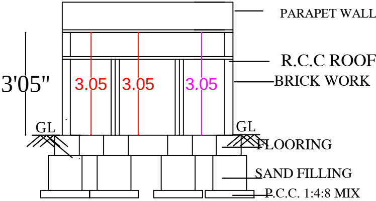
SECTION ONAA // 9" // 1'3" // 1'6"
