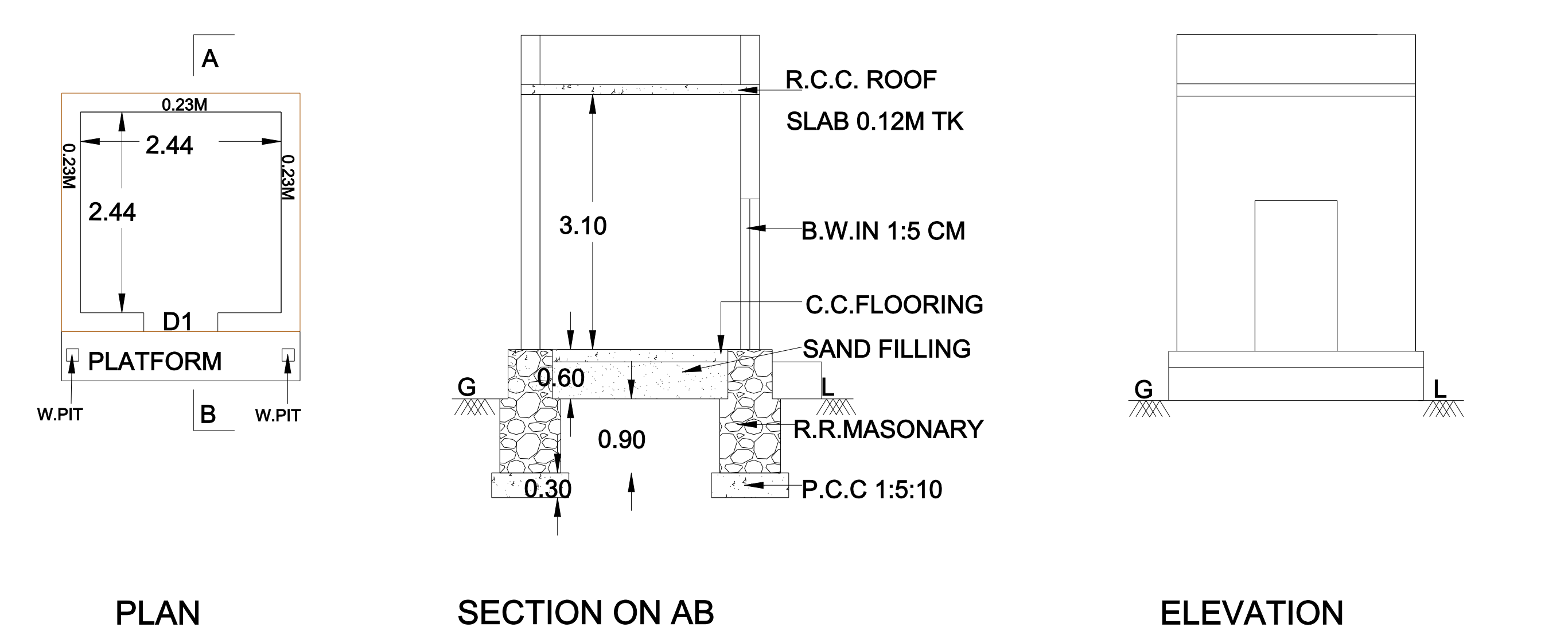
SULPHUR ROOM NO : 5
