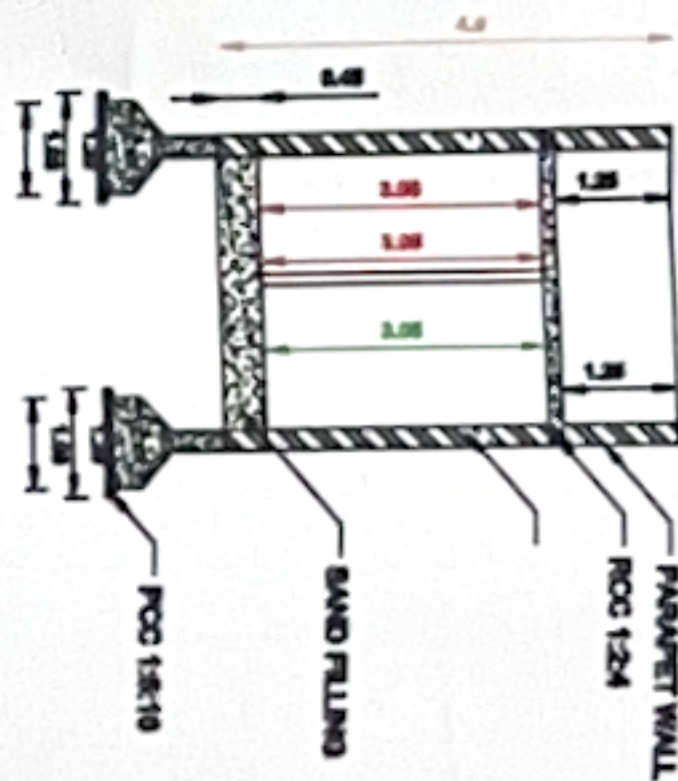
SECTION A-A'
