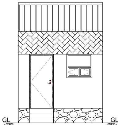
ELEVATION
