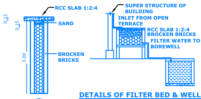
PERCOLATIONN PIT
