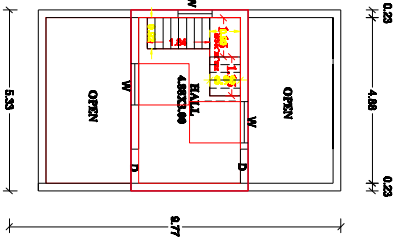
F.F. PLAN
