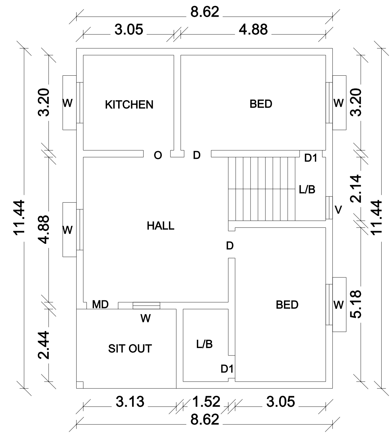
G.F PLAN
