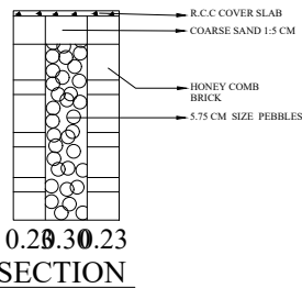
0.20.30.23 SECTION PLAN
