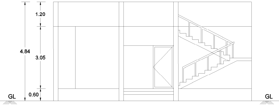
ELEVATION - A ELEVATION
