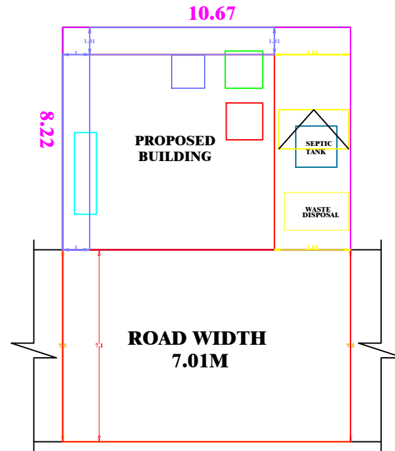
SITE PLAN 1:100
