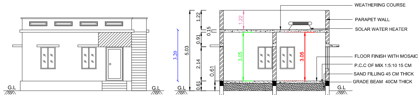
ELEVATION
