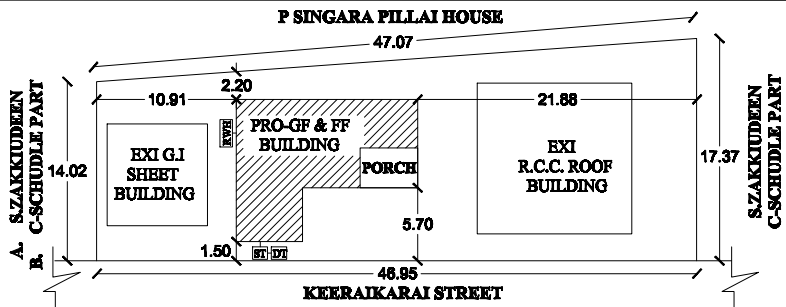
SITE PLAN SCALE 1:400
