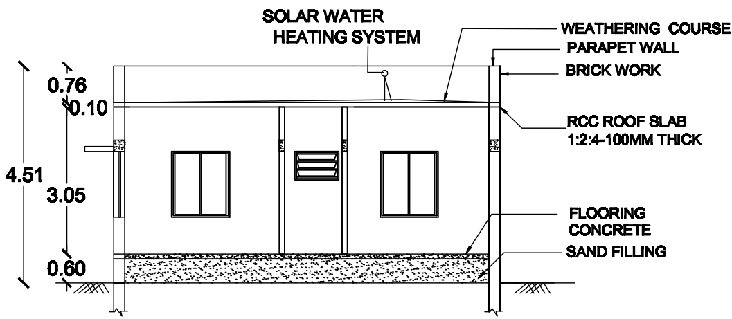
SECTION - 'RM'
