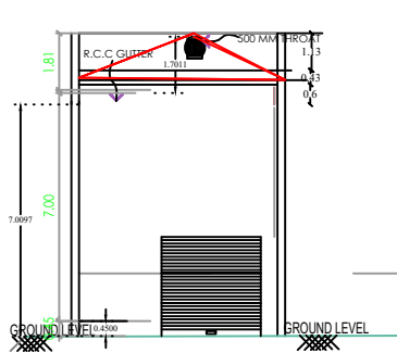
ELEVATION AB
