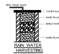
RAIN WATER HARVESTING R.W.H.
