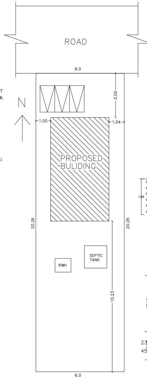
SITE PLAN 1:100
