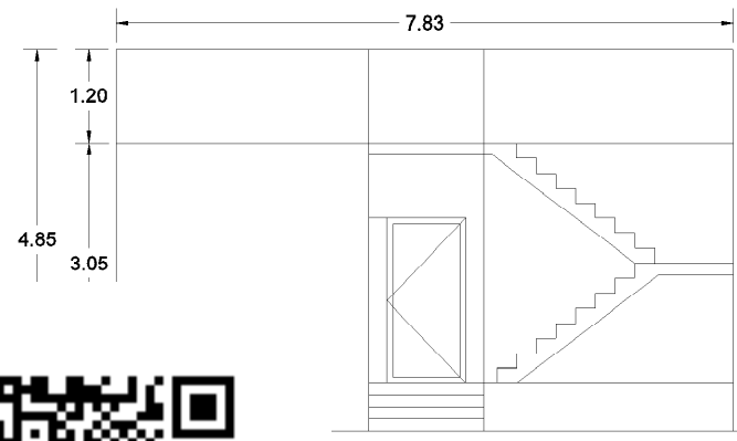
ELEVATION - A ELEVATION
