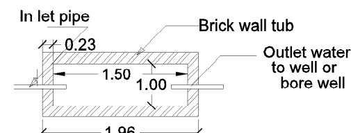
ELEVATION - A ELEVATION
