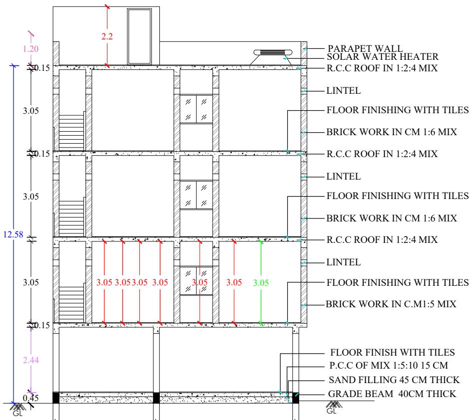
SECTION A-A1
