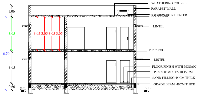
SECTION -AB
