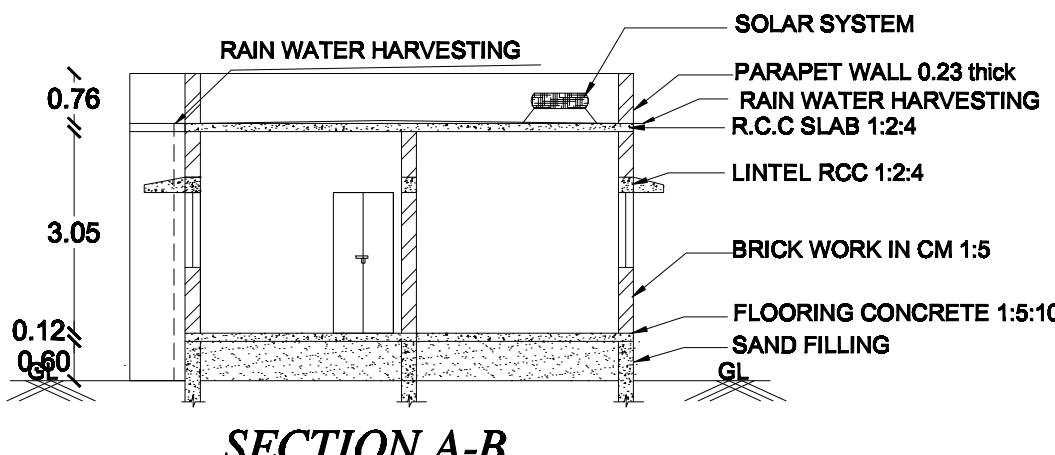
SECTION A-B
