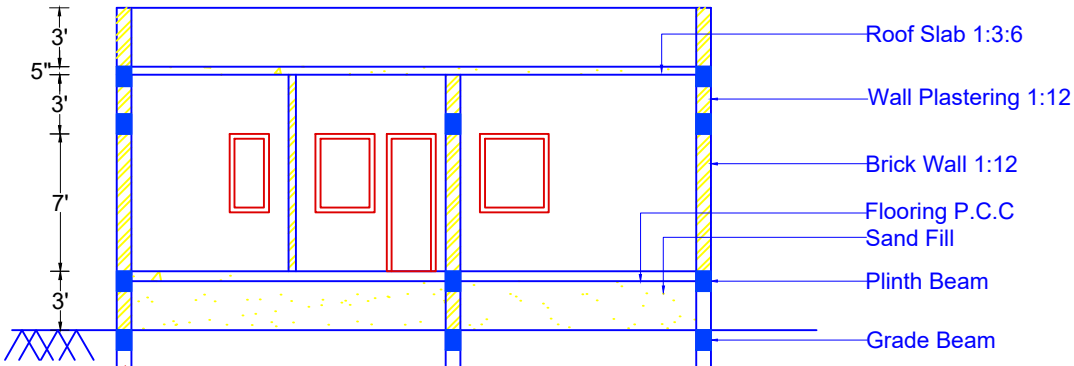
Section A-A
