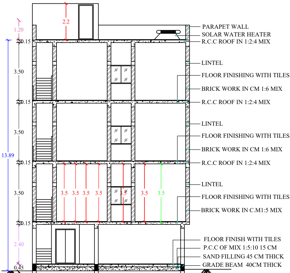
SECTION A-A1
