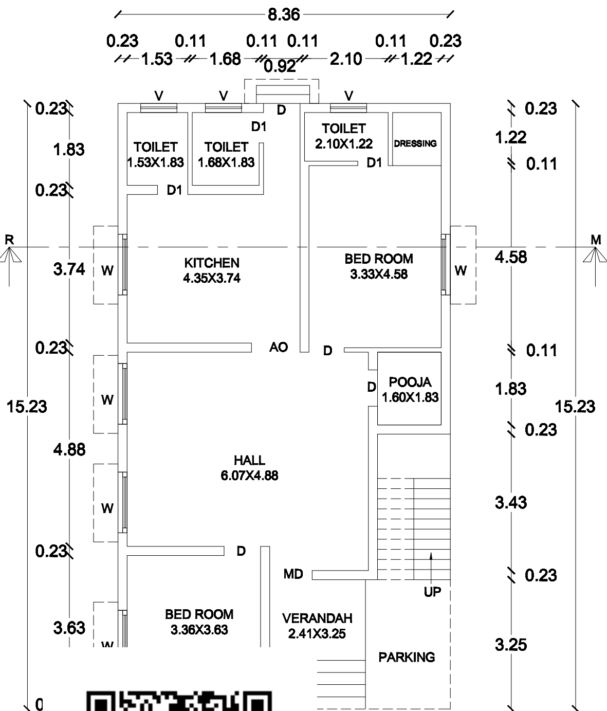
DOOR PLAN
