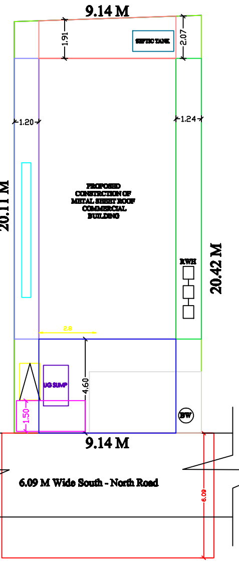
SITE PLAN 1:100
