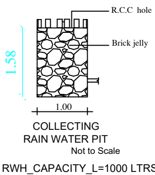
RWH_CAPACITY_L=1000 LTRS
