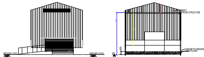
ELEVATION
