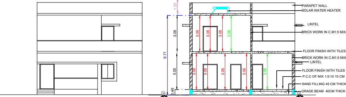
ELEVATION
