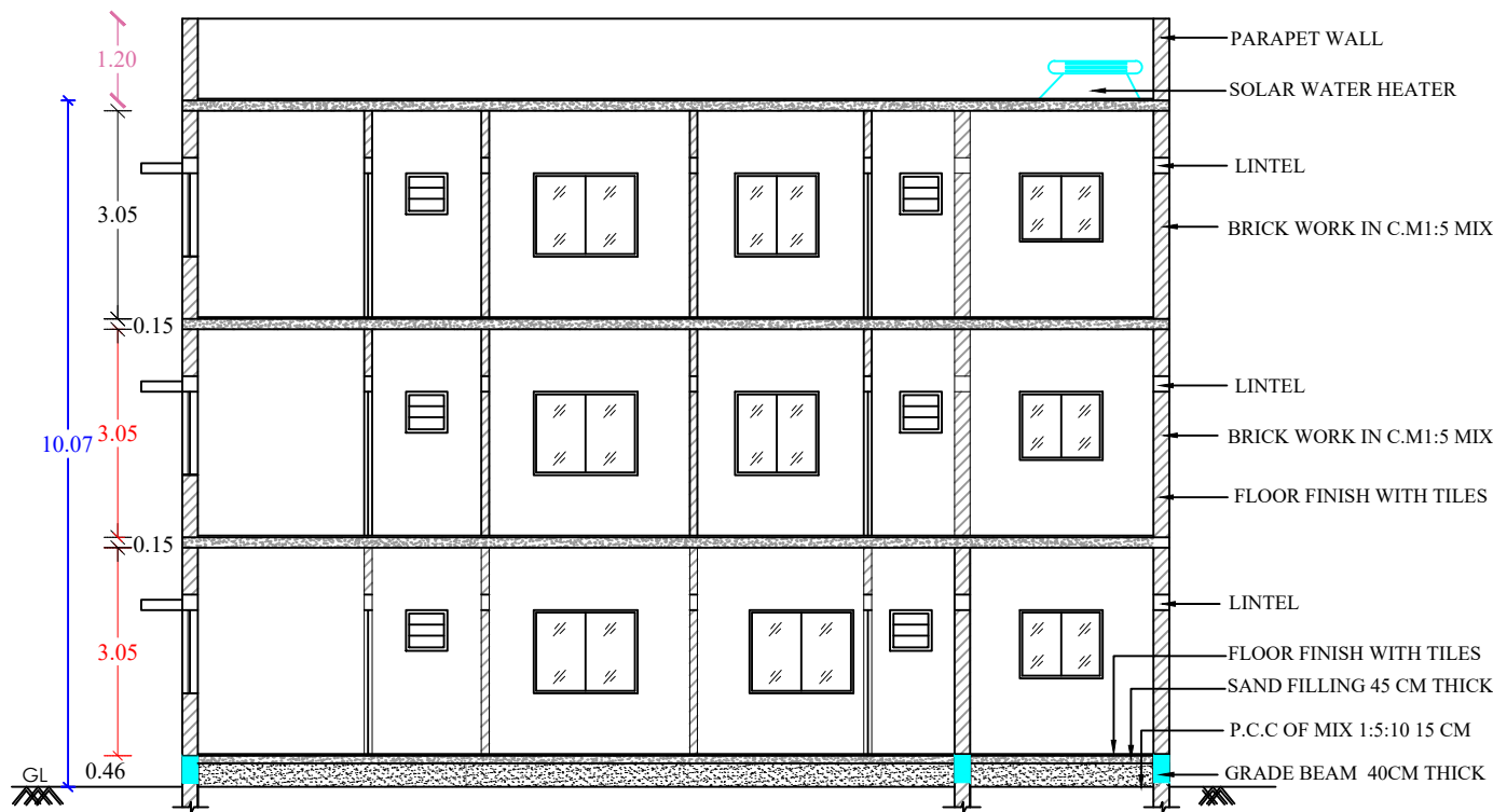
SECTION A-A1
